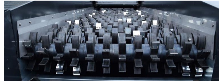
Grobsiebdeck bei Komtech Multistar One
