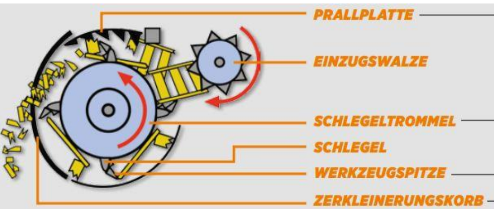
Funktionsaufbau Doppstadt AK-Serie
